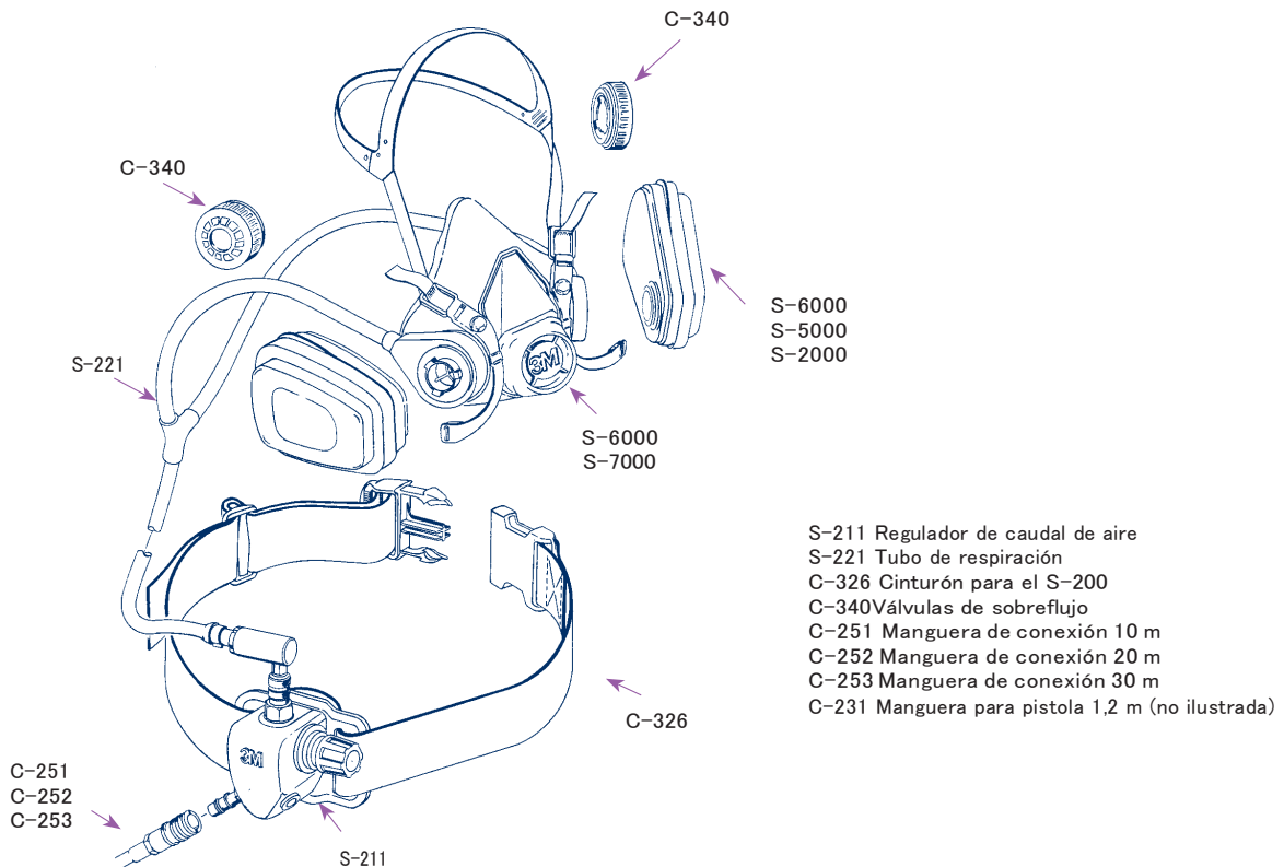
Equipos de suministro de aire comprimido 3M Serie 200
