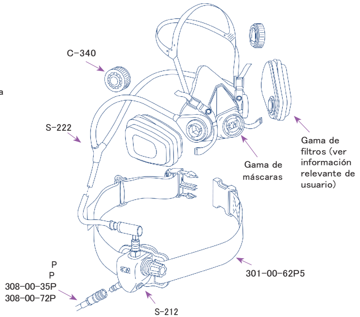
Equipos de suministro de aire comprimido 3M Serie 200
